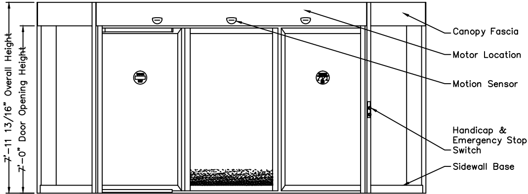
① Elevation
