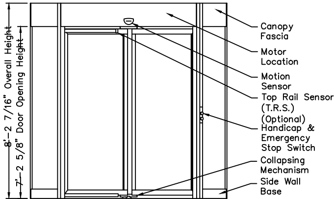
① Elevation
